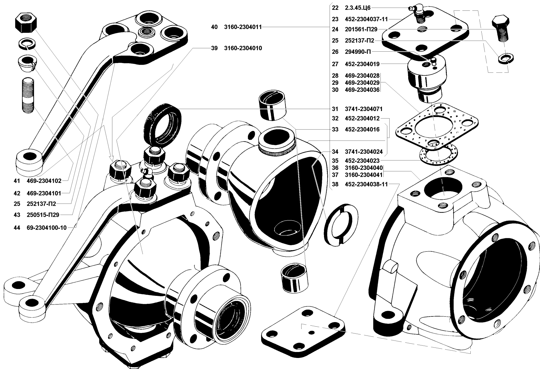
Рис. 57. Кулаки поворотные (2304)/2
